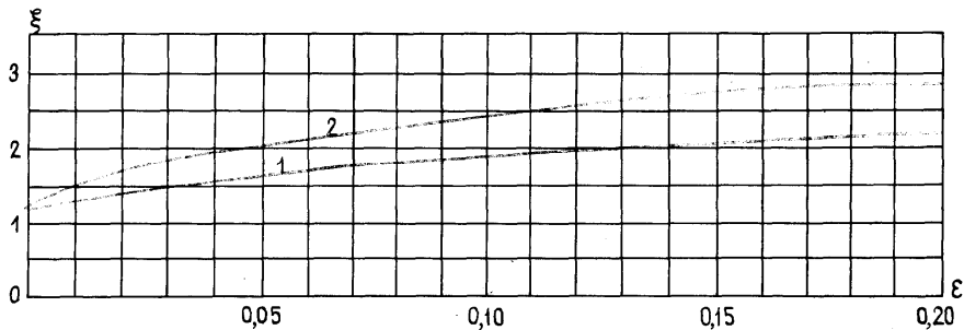
Черт. 2. Коэффициенты динамичности
